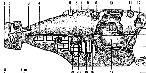
Καταδύμενο SM 97: 1. προφύσιο 2. κύρια έλικα 3. κινητήρας κατεύθυνσης προφύσιου 4. θάλαμος συσσωρευτών 5. υποβρύχιο τηλεφώνιο 6. κεραία ραδιοτηλεφώνου 7. αναλάμπων φανός (φλας) 8. δακτύλιος πόντισης 9. κατακόρυφη έλικα 10. καταπακτή σφαιρικού θαλάμου 11. εγκάρσια έλικα 12. πανοραμικός ηχοβολιστής (σόναρ) 13. φωτογραφική μηχανή 14. φινιστρίνι 15. θραχίονας τηλεσυλλληπτικός 16. κάλαθος 17. θάλαμος ενδιάτησης (σφαίρα πιανίου) 18. ρυθμιστής 19. δεξαμενή μεταλλικού έρματος 20. απόθεμα οξυγόνου 21. θήκη ηλεκτρονικού εξοπλισμού.
